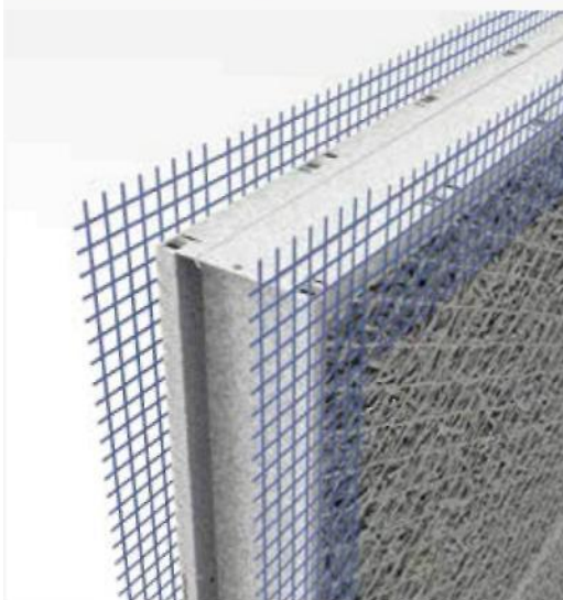
3. Задня профільована стійка. Утримує штукатурку всередині стійки й прикріплює всю структуру до стіни, в той час як зовнішня сітка запобігає утворенню нерівностей..
