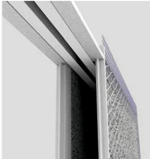
1. Профіль для вирівнювання з стіною. Зміцнює жорсткість направляючих, захищає їх від цементного розчину й утримує товщину стін.
